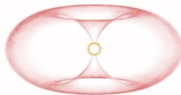
Solar Torus
