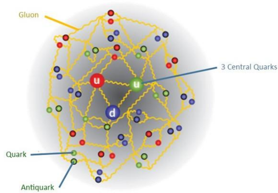
Quark/antiquark subatomic particle
