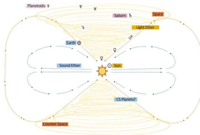
The Solar Torus Vortexes
