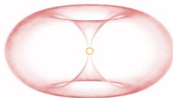
Solar torus
